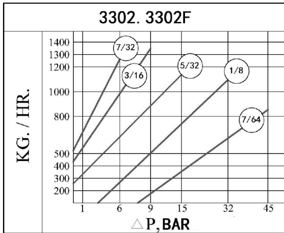
排量-冷凝水(Kg/h)(圆圈内为孔口直径)
