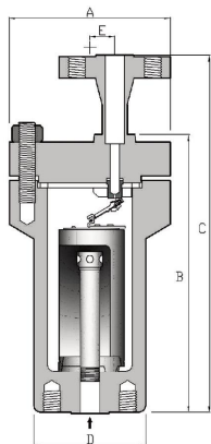
IB500,600 系列 尺寸, 最高操作压力与重量 (近似) -mm/bar/kg
