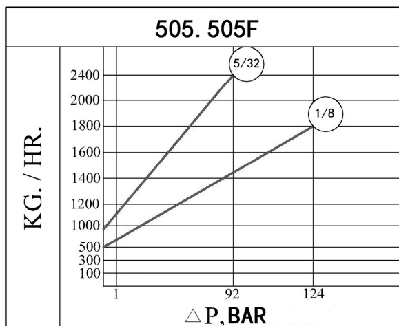
排量-冷凝水(Kg/h)(圆圈内为孔口直径)
